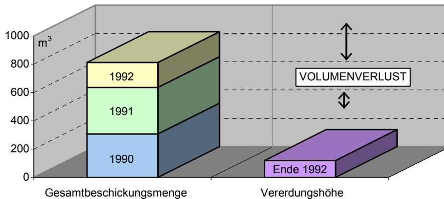
Abb.27: Volumensverringerng im Klärschlammbecken in Heiligenkreuz/Wassen
