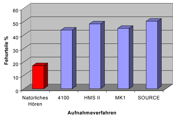
Abb. 4 Median-plane errors
